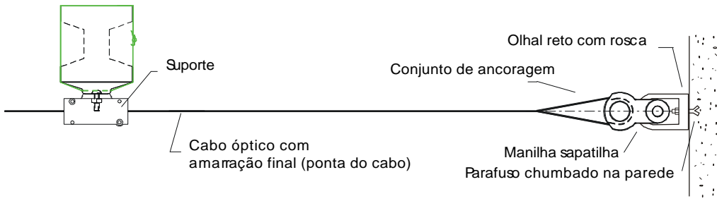
Ancoragem na parede com olhal reto e parafuso chumbado na parede
