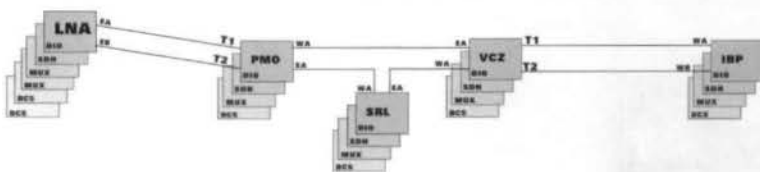
DIAGRAMA DE INTERCONEXÃO ÓPTICA LONDRINA
